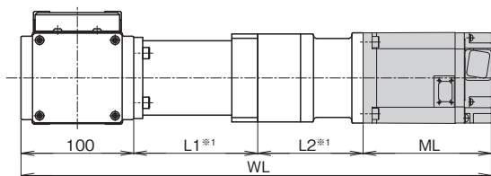
A矢視
